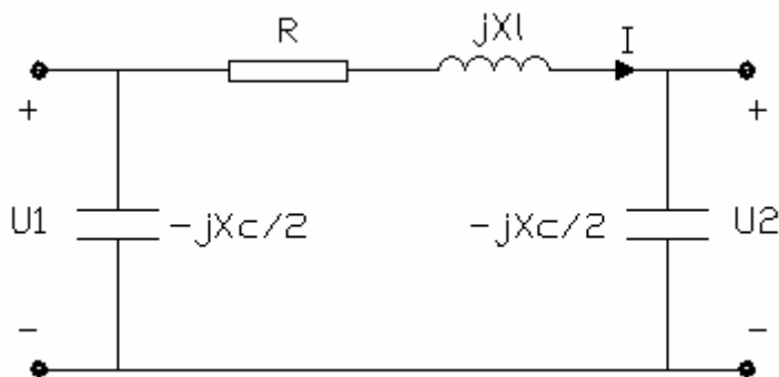
Figur 16. Det så kallade \pi -schemat för modellering av kabel.
