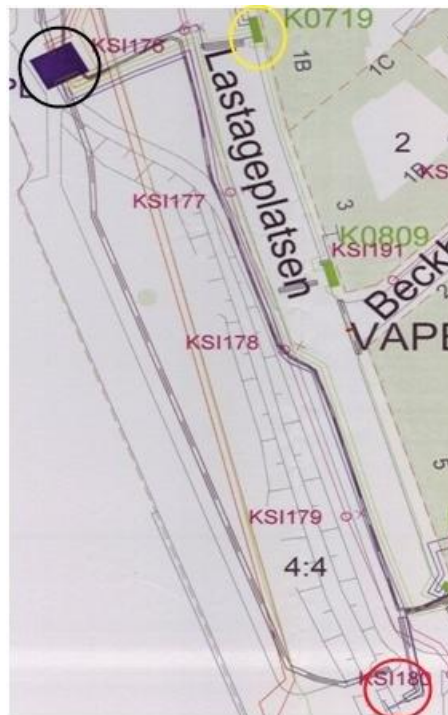
Figur 50. Områdeskarta, nätstationen finns längst upp till vänster (svart ring), frekvensomriktaren längst ner till höger (röd ring) och mätarrum finns till vänster om den gula markeringen. Större karta finns i bilaga B.
