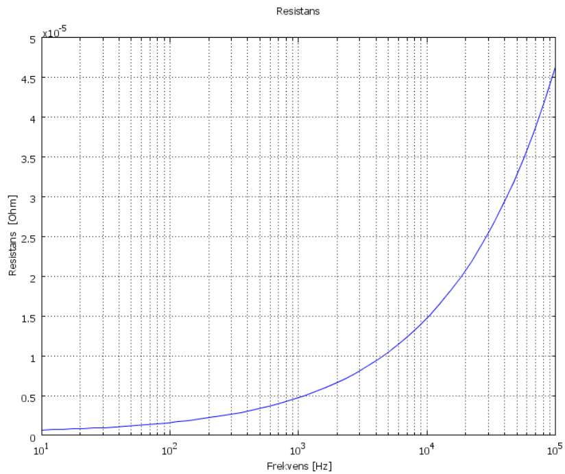
Figur 45. Resistansen beroende på frekvensen för modellen med en kardel, figur till höger.
