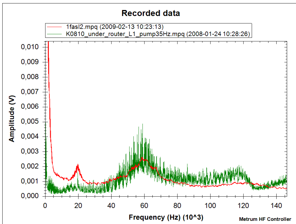
Figur 48. Jämförelse mellan den första mätningen (grön) och den andra utvärderande mätningen (röd).
