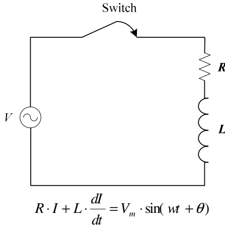
fig. 8. RL-circuit
