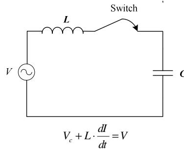
fig. 10. LC circuit
