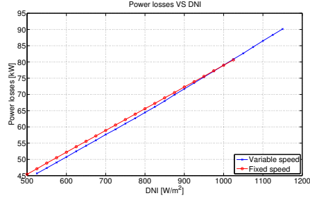
(d) Losses in CSP stirling power plant
