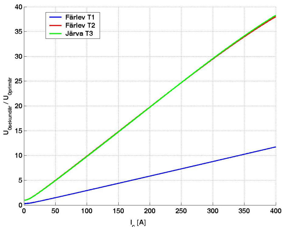
Figur 25: Simulerad nollföljdsspänningskvot mellan sekundärsida och primärsida med kontinuerligt avstämt nät.
