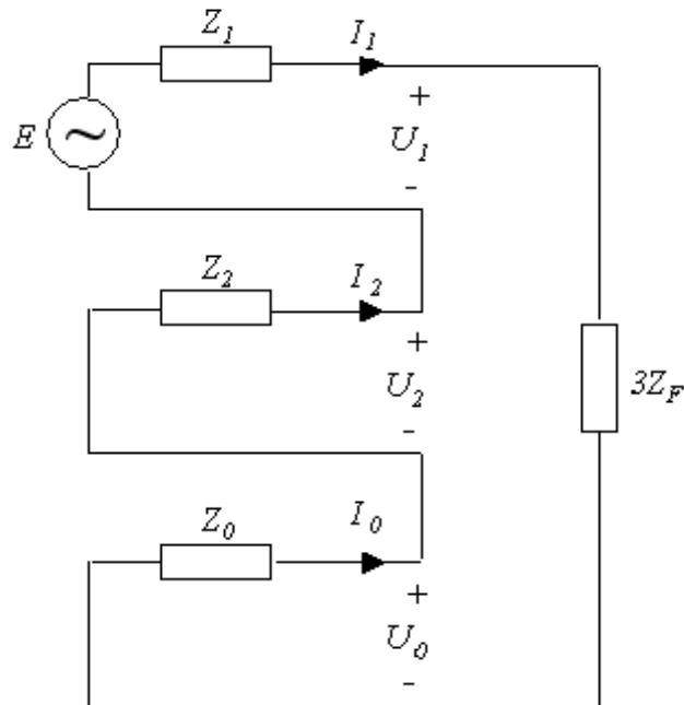
Figur 5: Sekvensnätskoppling för ett enfasfel med felimpedans Z_F .
