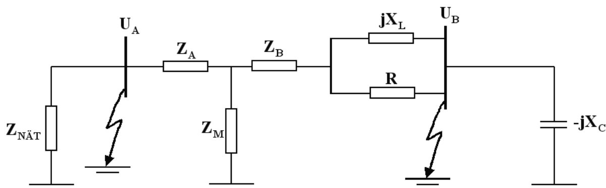
Figur 24: Resonanskrets i nollföljd. Fel vid U_A medför serieresonans och vid U_B parallellresonans.
