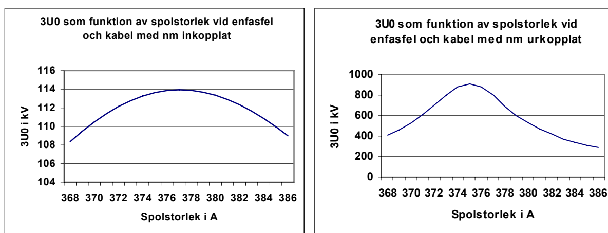
Figur 23: Inverkan av snedavstämning vid simulerat fel primärt på Färlev A vid kablfierat 40 kV nät.
