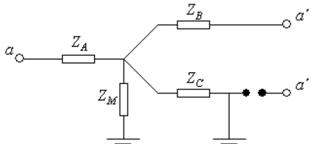
Figur 13: Nollföljdsmodell för en Y/y/ \Delta -kopplad transformator.
