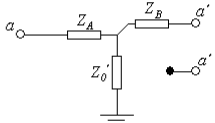
Figur 14: Förenklad nollföljdsmodell för en Y/Δ-kopplad transformator.
