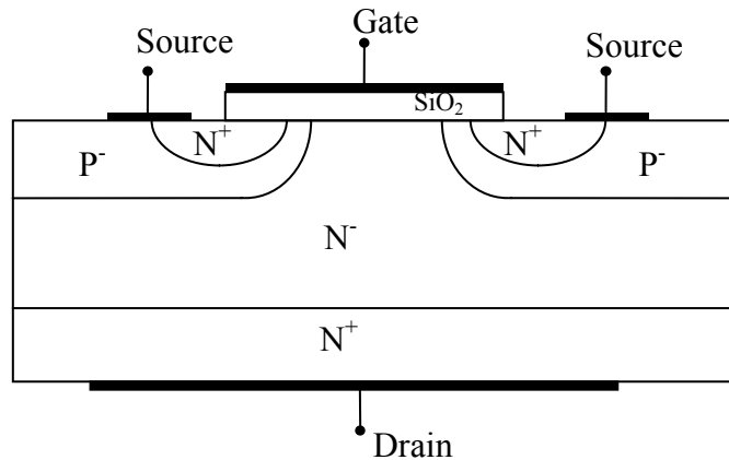
Figure 47. DMOSFET.
