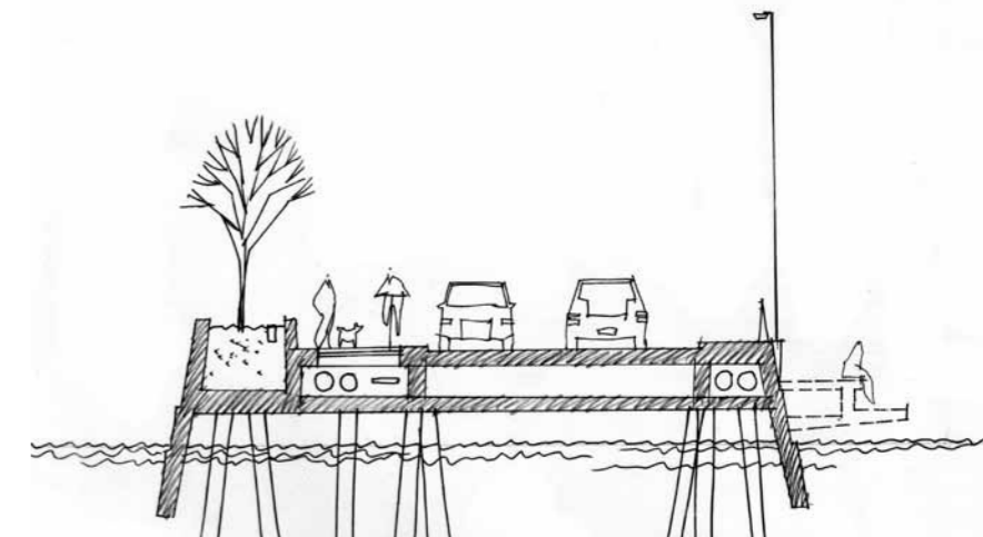
Sektion genom grundlagt pir där det fasta gatunätet ligger
